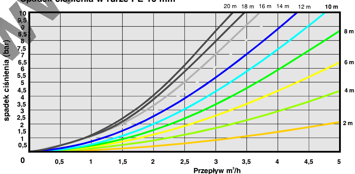
Spadek ciśnienia w rurze PE 16 mm
