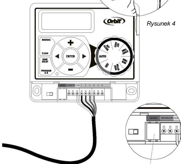
Rysunek 5 Podłącz transformator tutaj
